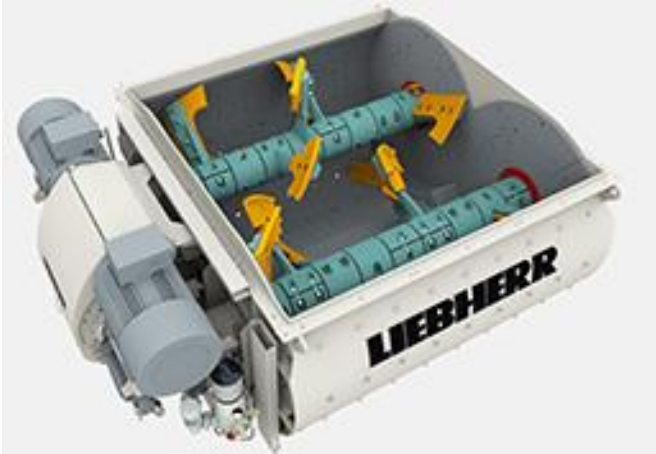
Mezclador Twin-Shaft DW 4.5
