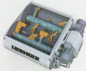
Doble Eje horizontal (Twin-shaft)
